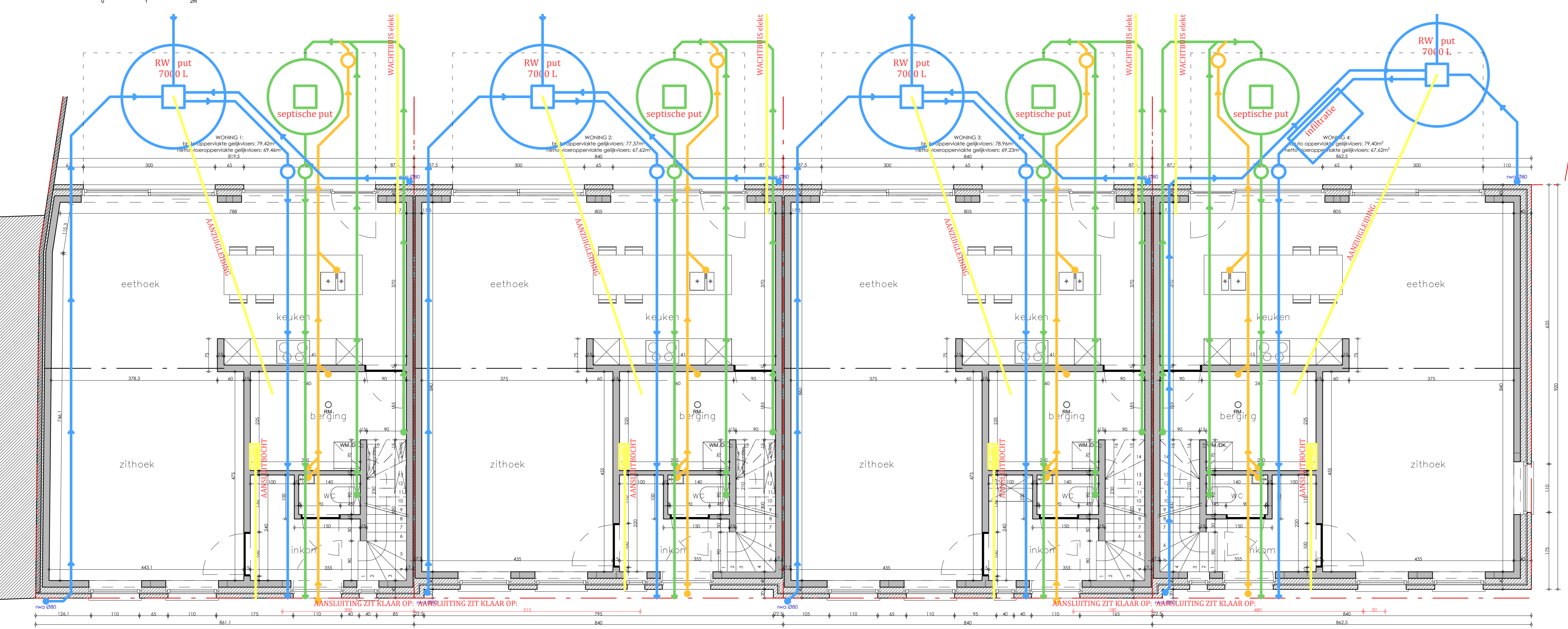
RIOLERING Schaal 1:50
