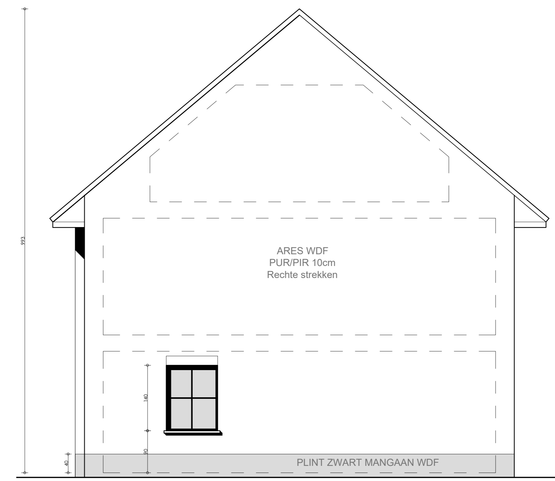
RECHTER ZIJGEVEL woning 4 Schaal 1:50
