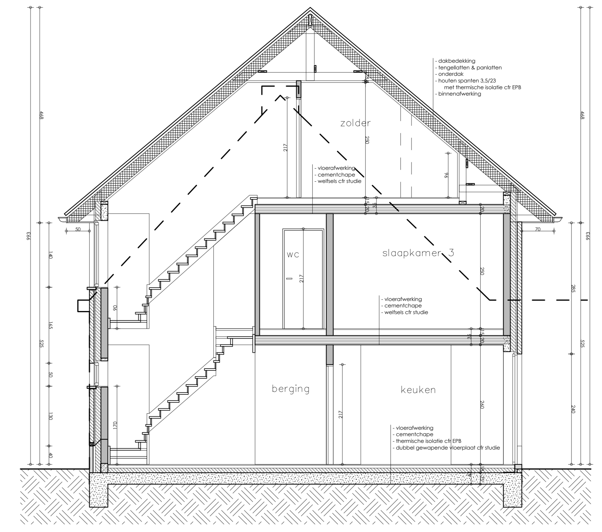
SNEDE AB Schaal 1:50
