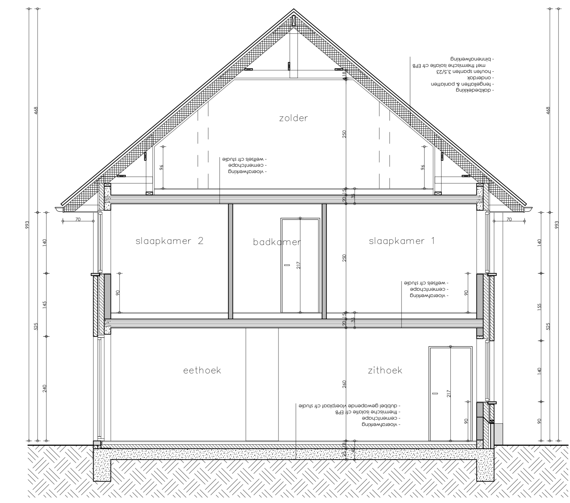
SNEDE CD Schaal 1:50
